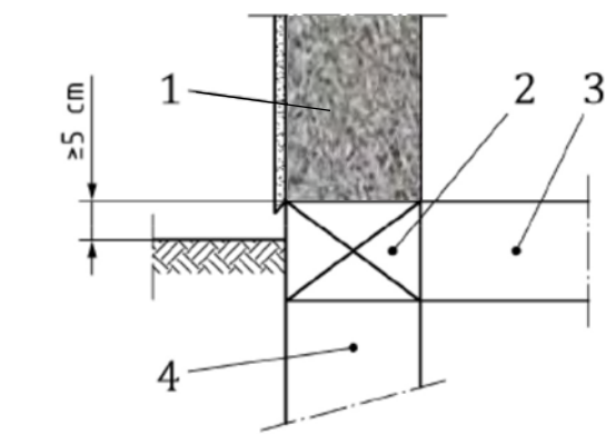
Figure A04 : Disposition anti-capillarité – solution 2 avec soubassement en béton armé
