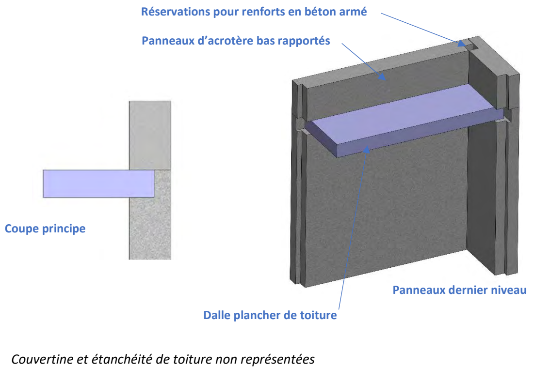
Figure A24-D : Acrotère bas rapporté sur dalle toiture
