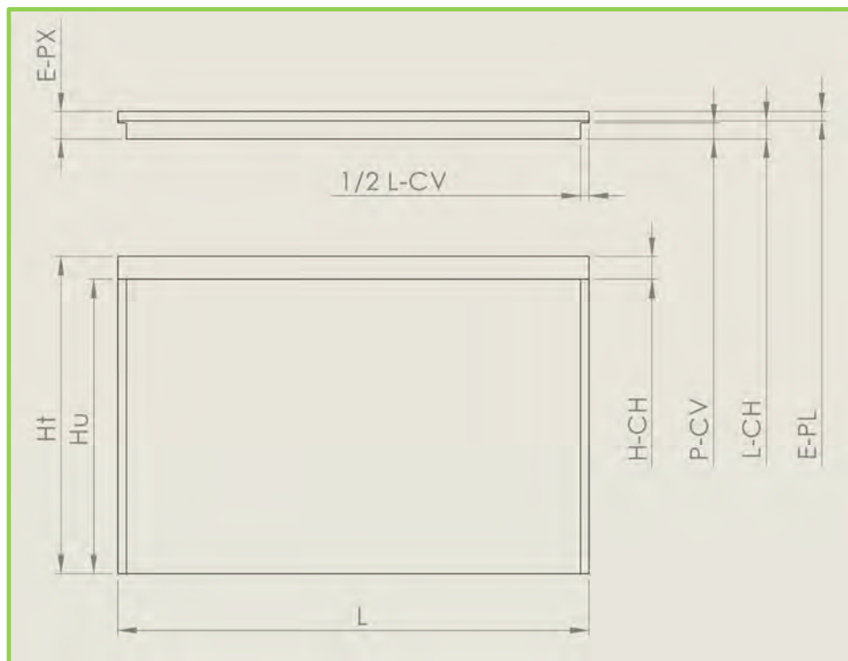
Figure 1B Dimensions limites pour un panneau plein
