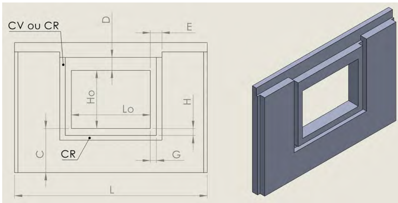
Figure 1M Généralités du positionnement des renforts ou chaînages d'ouvertures.
