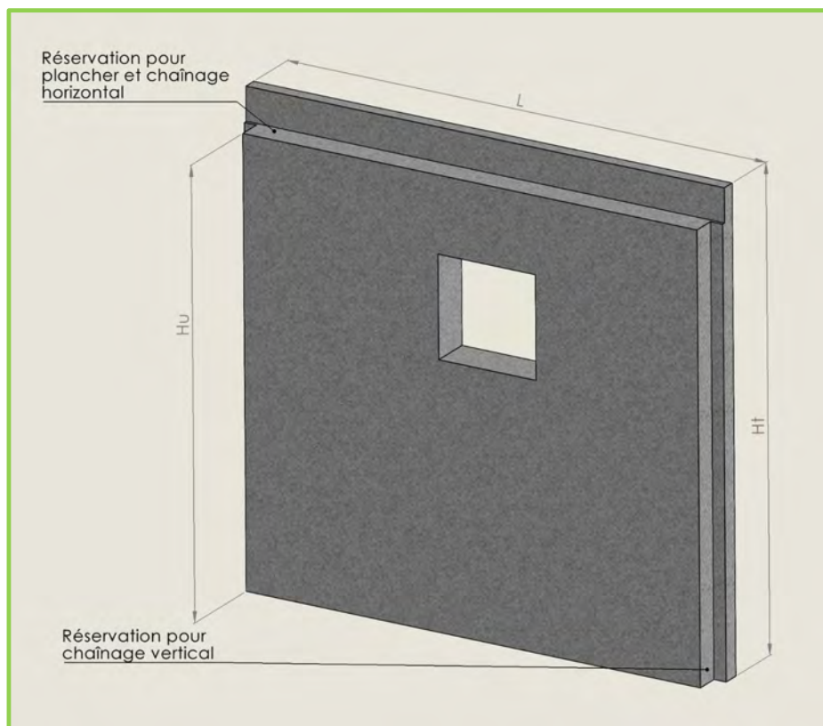
Figure 1A Vue globale d'un panneau en béton de bois CS2
