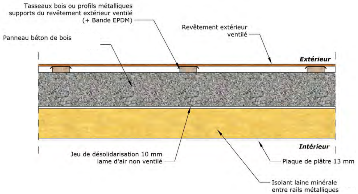
Figures A40 : Exemple partie courante Panneau avec bardages
