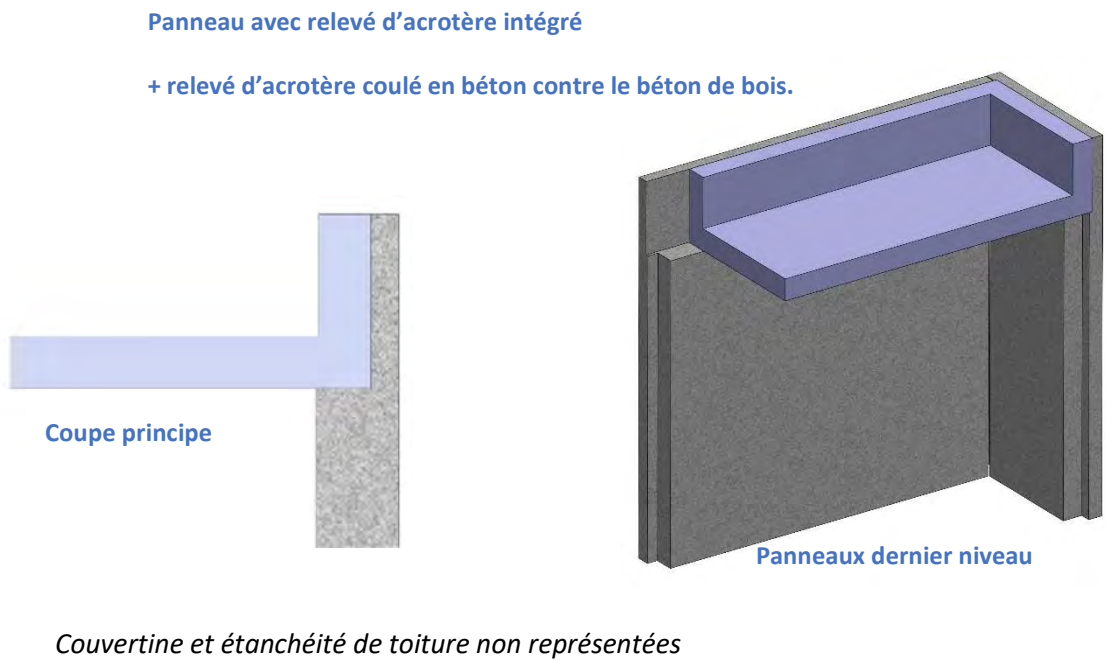
Figure A24-C : Acrotère bas mixte
