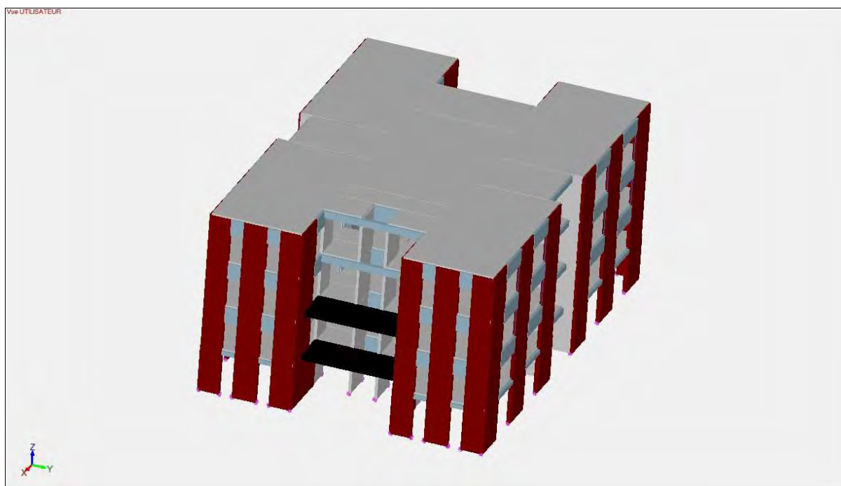
Fig. 14 – Modèle mixte (béton en gris et CS2 en rouge) - Axonomie 3
