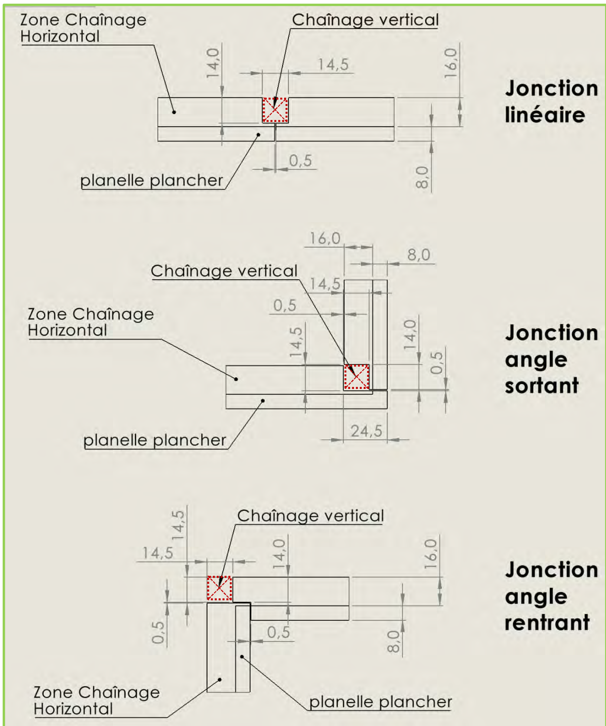
Figure 11 Détails jonctions de panneaux 24cm
