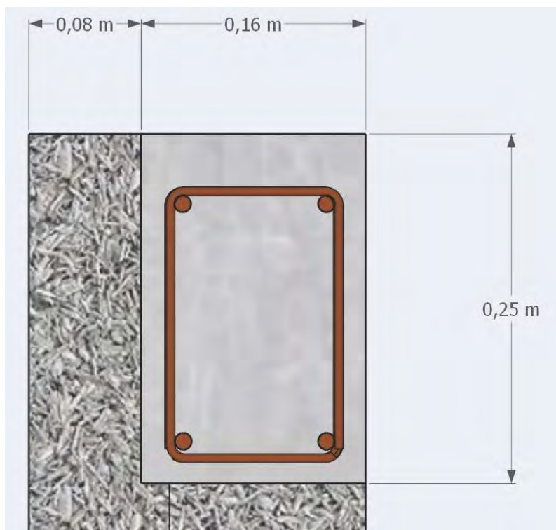
Figure A08 : Vue de principe en coupe d'un chaînage horizontal : Panneau de 24 cm d'épaisseur avec un plancher d'épaisseur 25 cm – chaînage régissant sur 2/3 de l'épaisseur du mur.
