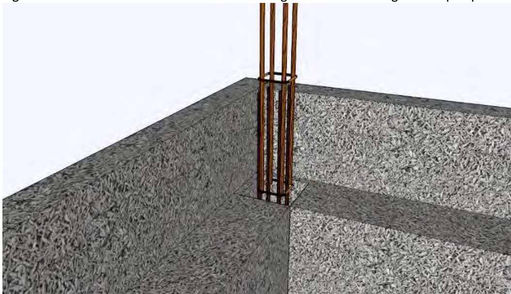
Figure A12 : Continuité des armatures de chaînages verticaux en angle – vue perspective
