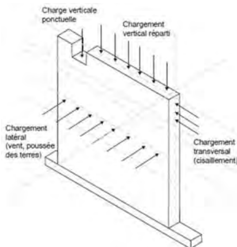
Figure A07-1 : Types de chargements appliqués sur les murs
