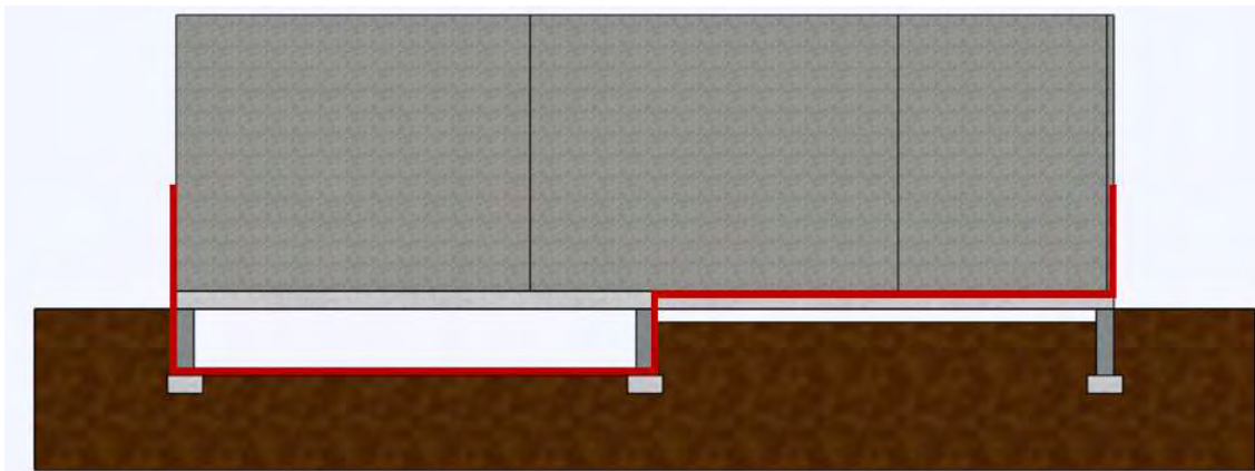
Figure A06 : Protection contre les termites – schéma de principe avec barrière continue
