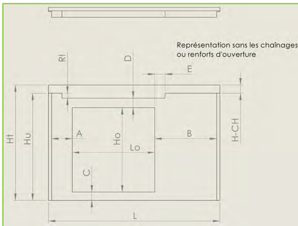
Figure 1C Dimensions limites pour un panneau avec ouverture Linteau en retombée de chaînage horizontal
