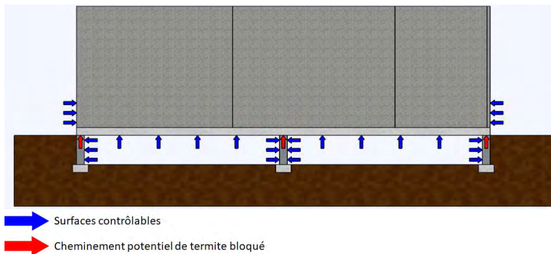
Figure A05 : Protection contre les termites – schéma de principe avec parois contrôlables
