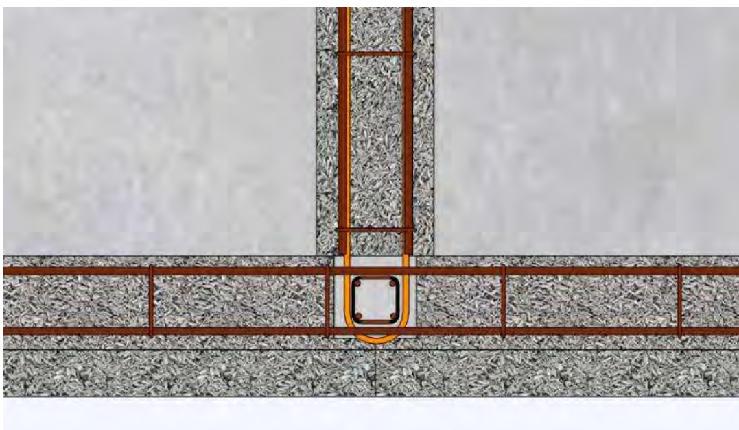
Figure A14 : Continuité des armatures de chaînages horizontaux avec boucles U – Liaison refend
