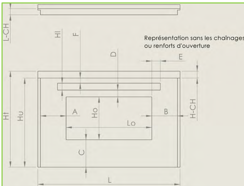
Figure 1D Dimensions limites pour un panneau avec ouverture Linteau intégré classique
