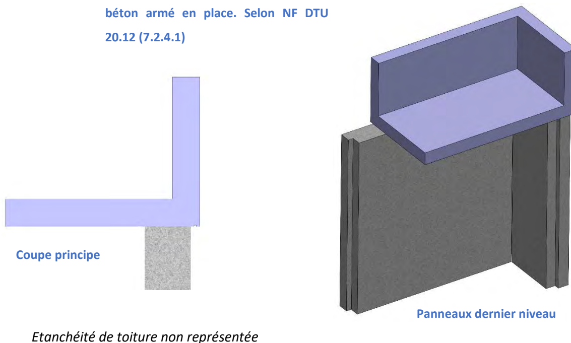
Figure A25-A : Acrotère haut coulé en place
